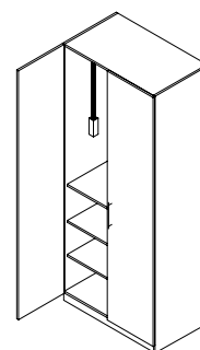
Skřín šatní, policová LS 100 V-P (100 x 242 x 60)
