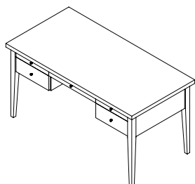
Stůl psací PS (150 × 75 × 75)
