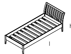
Postel jednolůžková LPR-1 s roštem (218 × 80 × 97)
