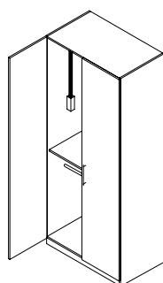
Skřín šatní LS 100 V - T (100 x 242 x 60)
