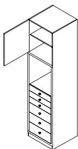
Skřín kombinovaná LS 60 - BZ (60 x 242 x 60)
