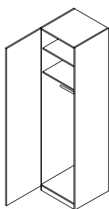
Skřín šatní LS 60 L-T (60 x 242 x 60)
