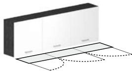
3 dveře VHO14 rozměr: 1800 x 600 x 300
